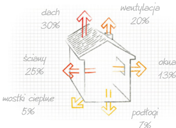
Rys.1 Straty ciepła w budynkach
