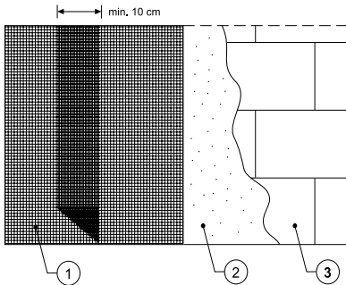
Rys.7 Montaż siatki na powierzchni ściany
